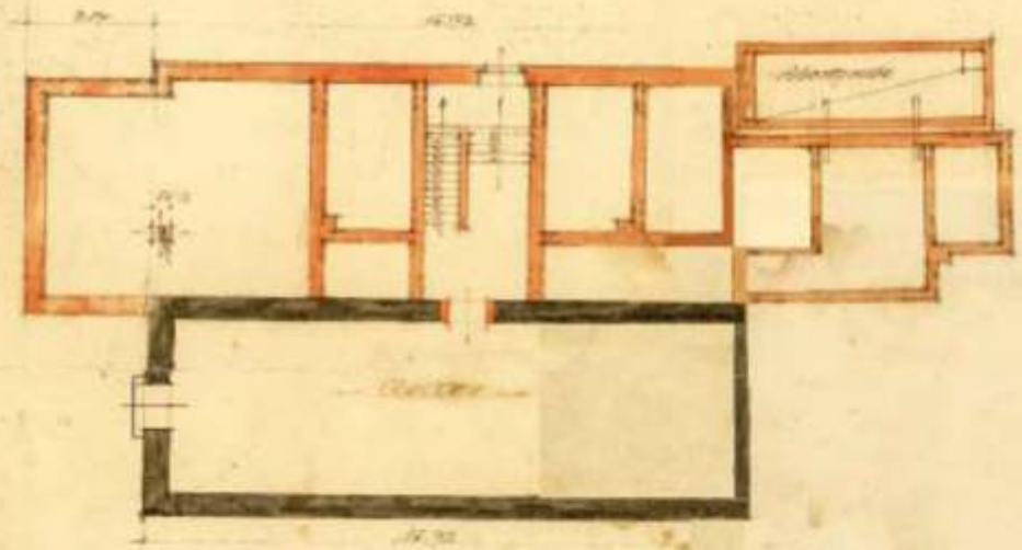
— Kellergeschoss —
