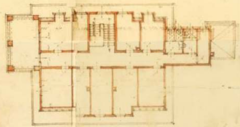
— Dachgeschoss —
